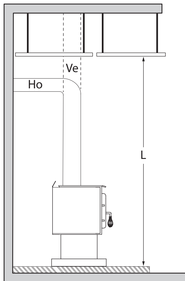
Figure 12: Dégagements - Plafond
