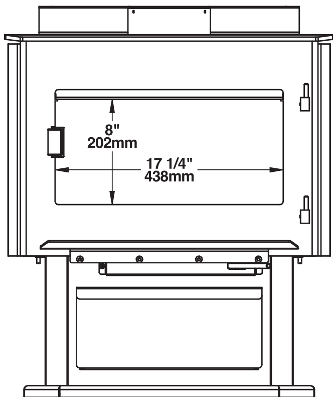
Figure 4: Ouverture de porte
