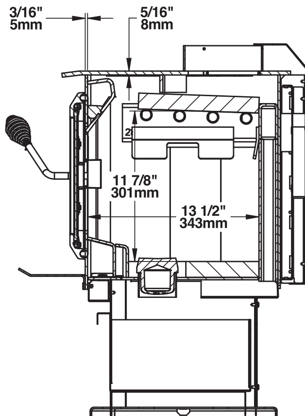
Figure 6: Vue de côté - chambre à combustion
