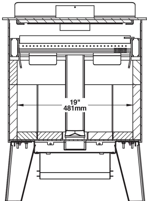
Figure 5: Vue de face - chambre à combustion
