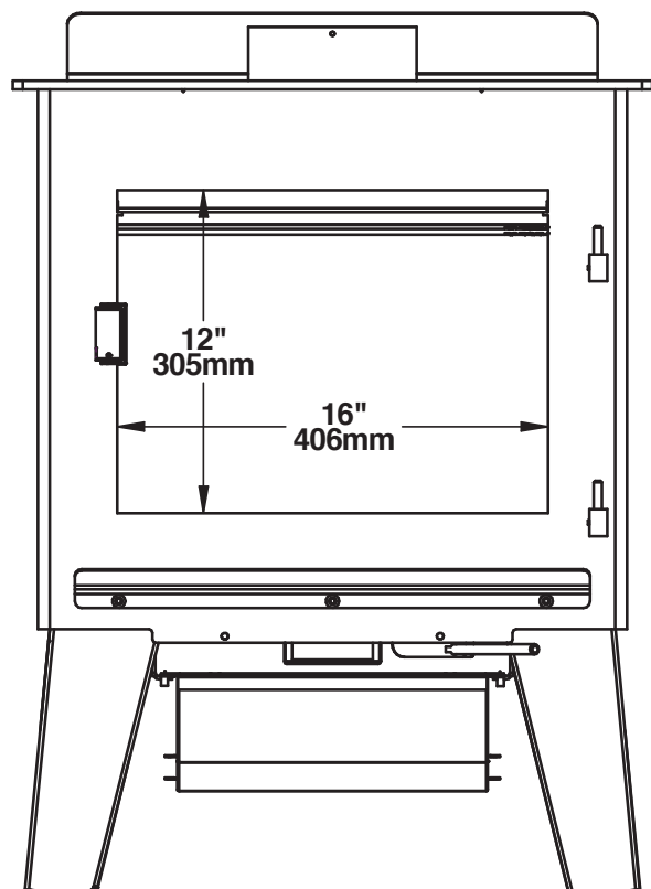
Figure 4: Ouverture de porte
