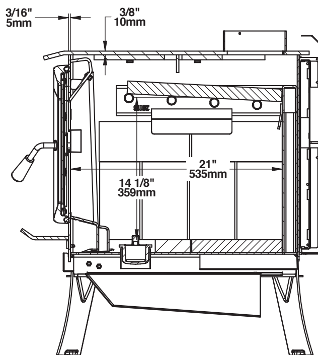
Figure 8: Vue de côté - chambre à combustion
