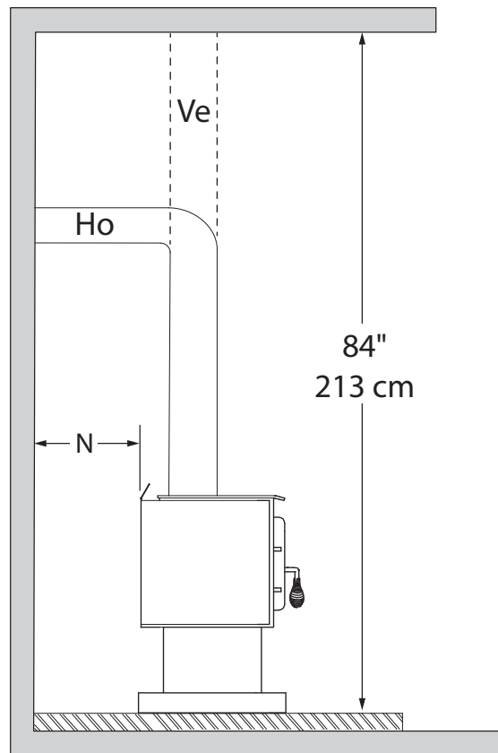
Figure 20: Dégagevements - Côté
