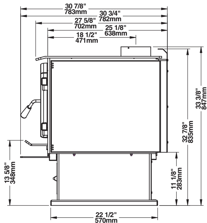
Figure 5: Vue de côté
