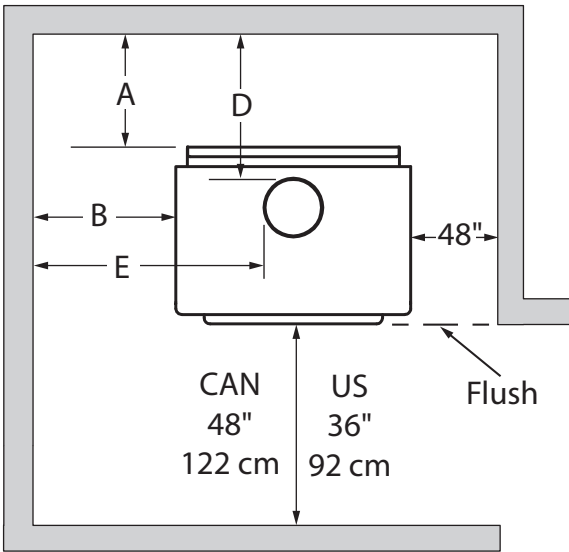
Figure 18: Dégagevements - Dessus
