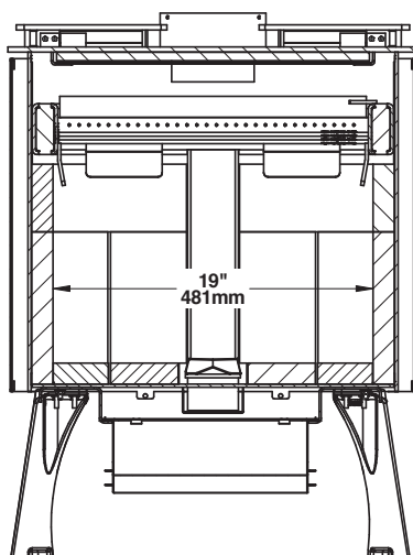
Chambre à combustion - Vue de face
