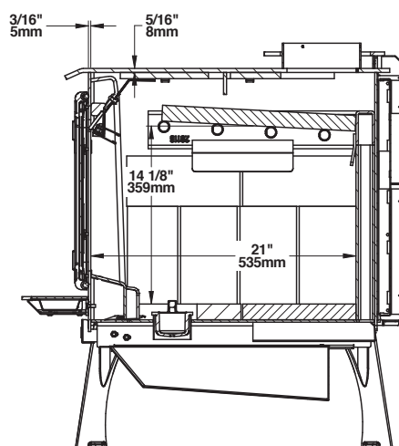
Chambre à combustion - Vue de côté
