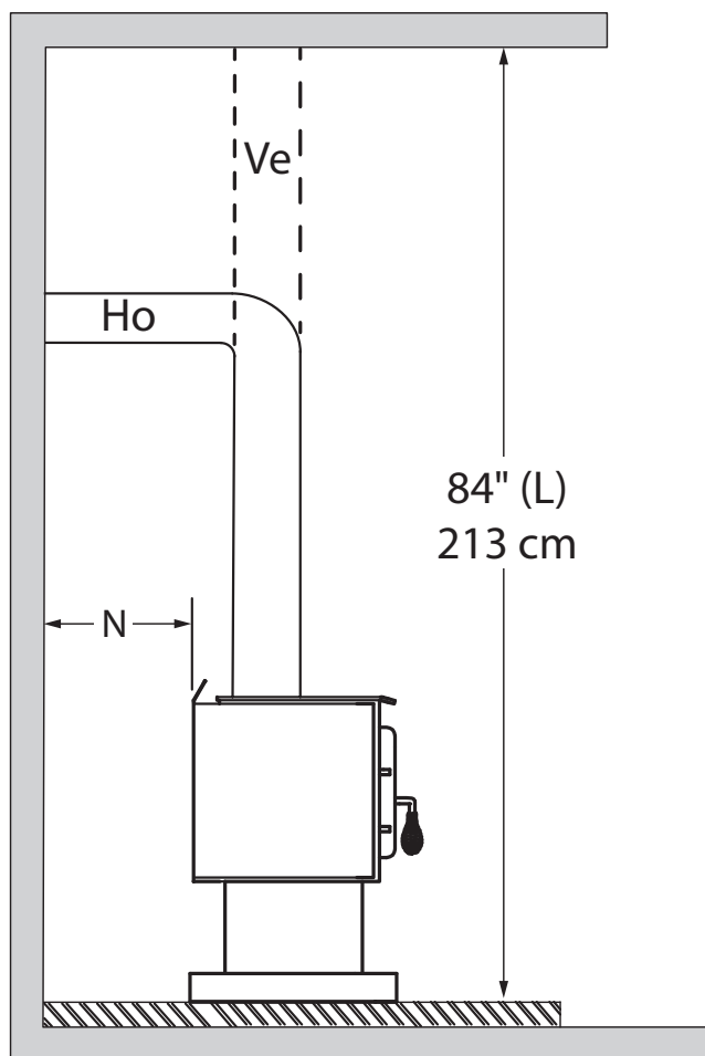
Figure 12: Développements - Côté
