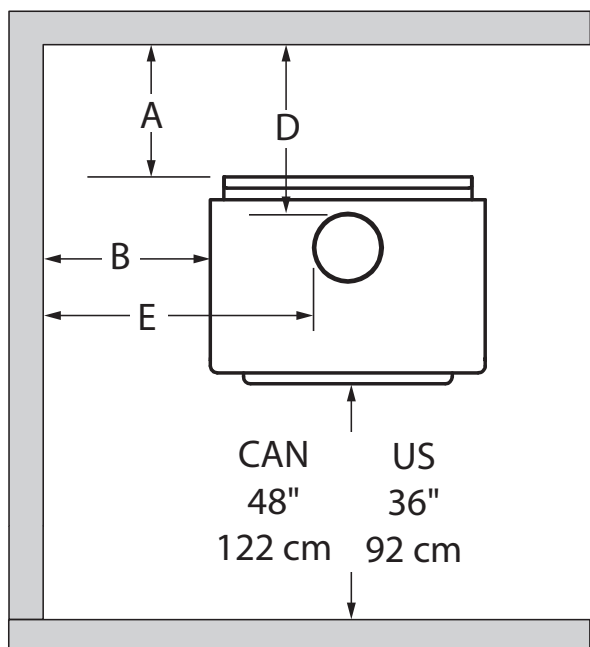
Figure 10: Développements - Dessus
