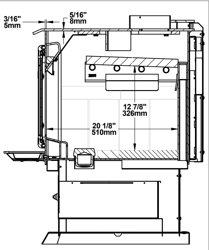
Figure 6: Vue de côté - chambre à combustion
