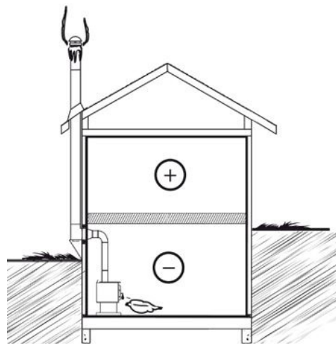
Figure 21: Conception de système inférieure
