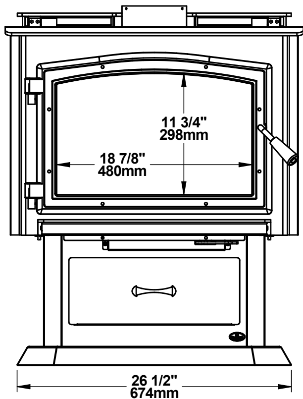
Figure 2: Vue de face
