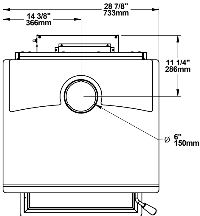
Figure 1: Vue de dessus
