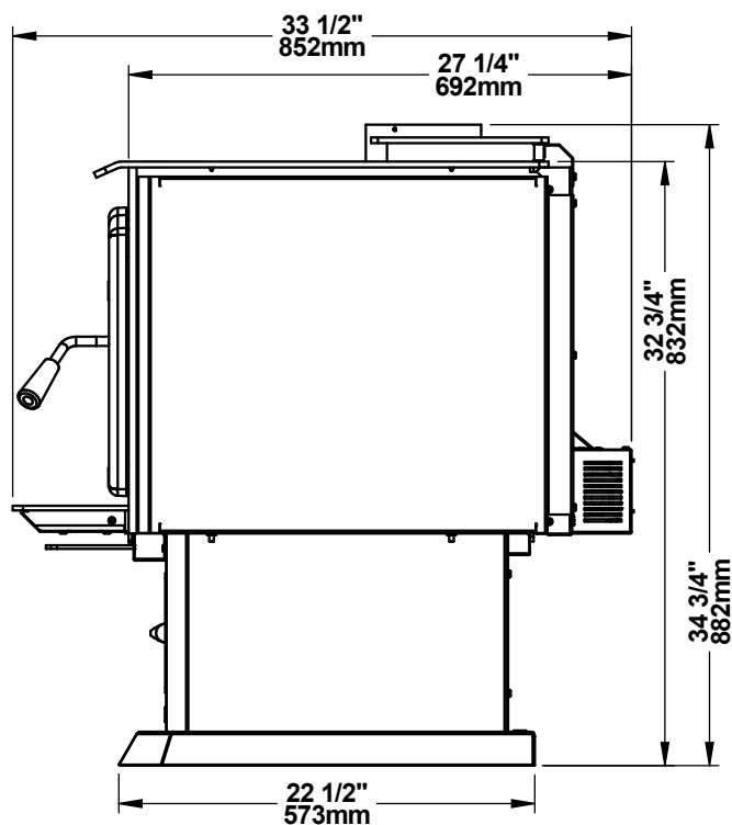
Figure 3: Vue de côté
