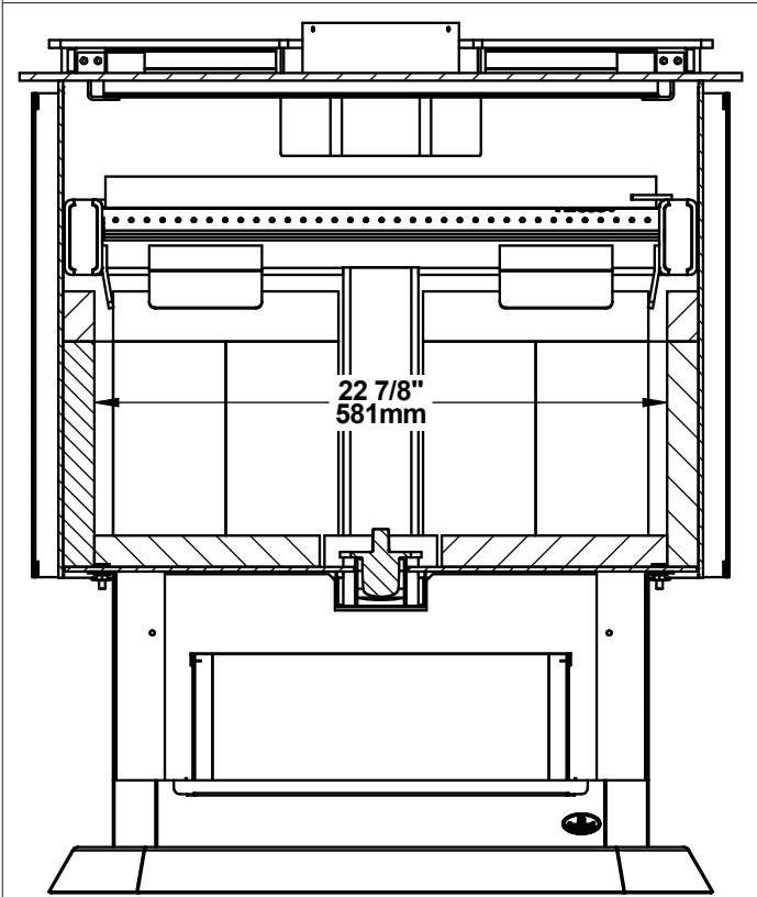
Figure 5: Vue de face - chambre à combustion
