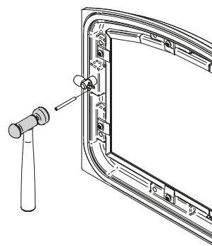
Figure 10: Installation de la goupille de retenue
