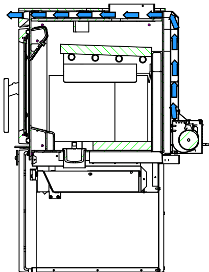
Figure 8: Circulation de l'air
