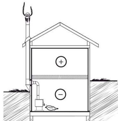
Figure 15: Conception de système à éviter
