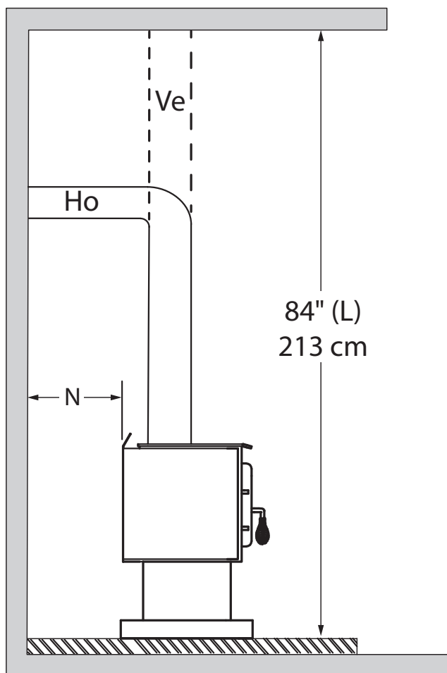
Figure 12: Développements - Côté
