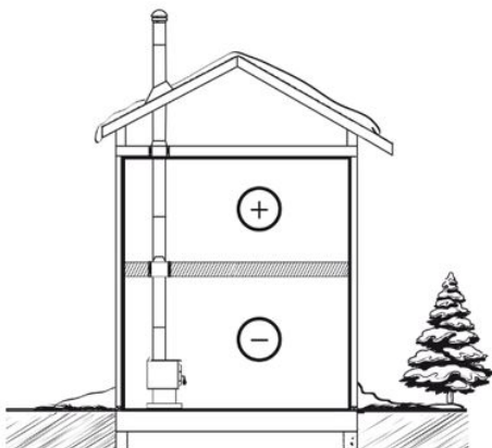
Figure 14: Bonne conception du système
