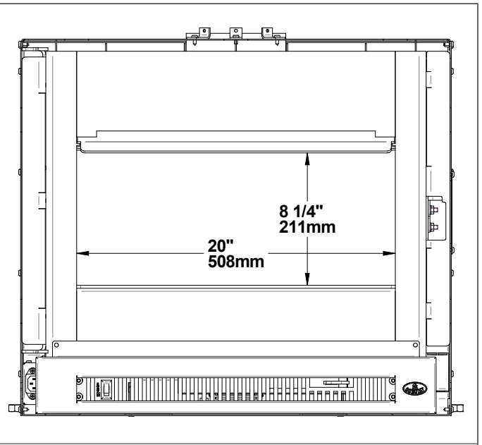
Figure 2: Ouverture de porte
