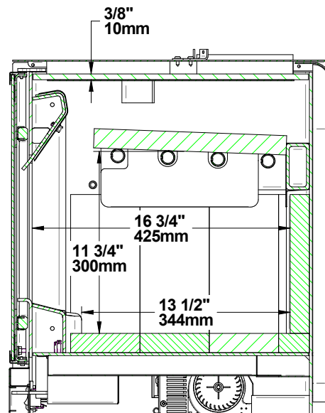
Figure 6: Vue de côté - Chambre à combustion
