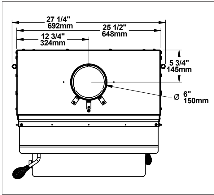
Figure 1: Vue de dessus
