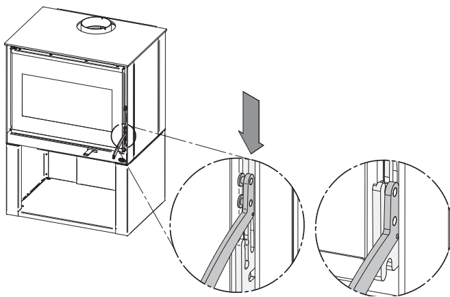
Figure 8: Ouverture à droite de l'encastrable
