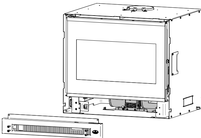
Figure 10: Emplacement du ventilateur
