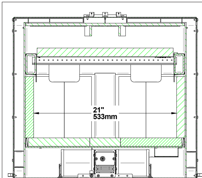
Figure 5: Vue de face - Chambre à combustion
