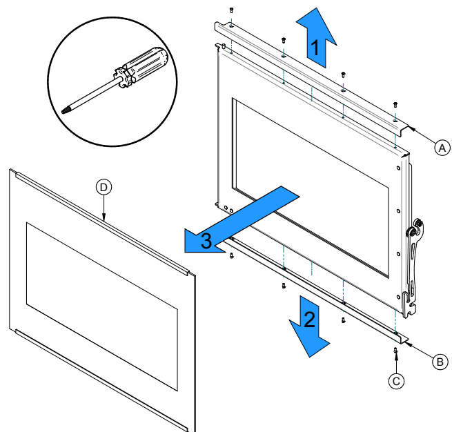
Figure 13: Remplacement la vitre
