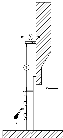
Figure 15: Dégagement de la tablette
