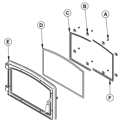
Figure 13: Remplacement de la vitre
