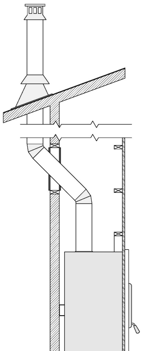
Installation avec déviation extérieure
